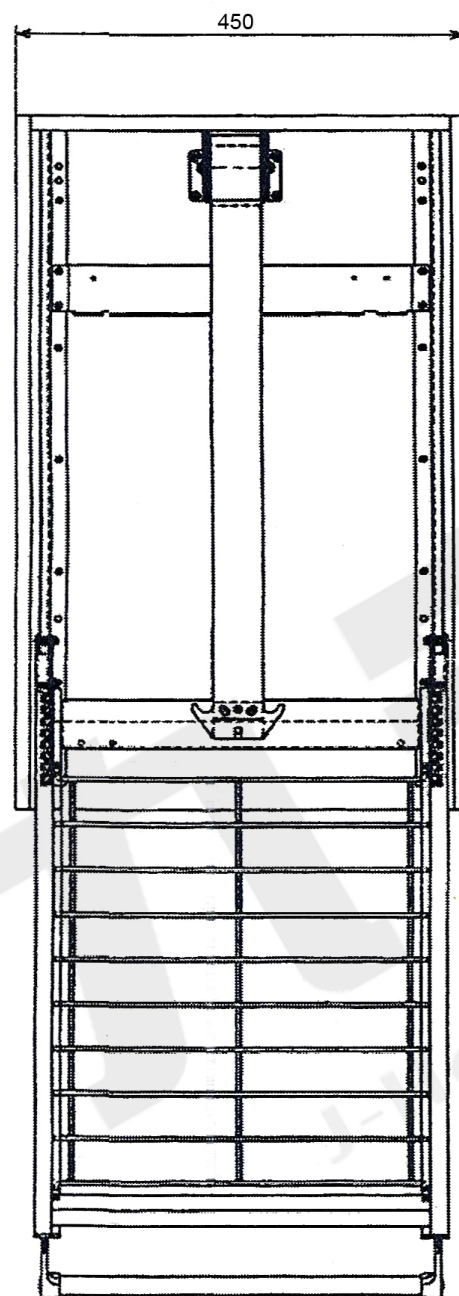
WP.693045日本升降拉架組-下降最低位置
