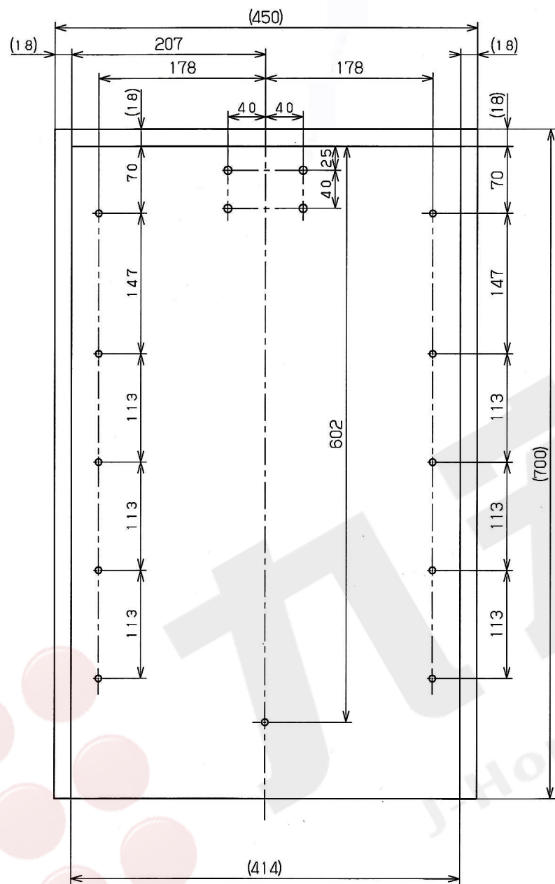
WP.693045日本升降拉架組-孔位圖
