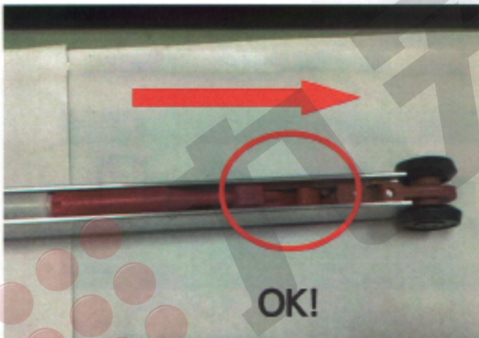
將塑膠件移至此位置
