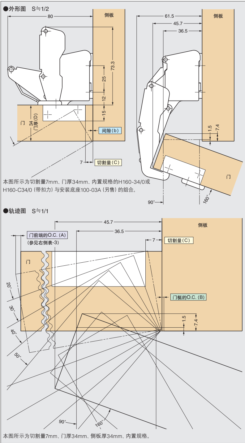
■切割量 (C) 与门框间隙 (b) 的关系 表-1
