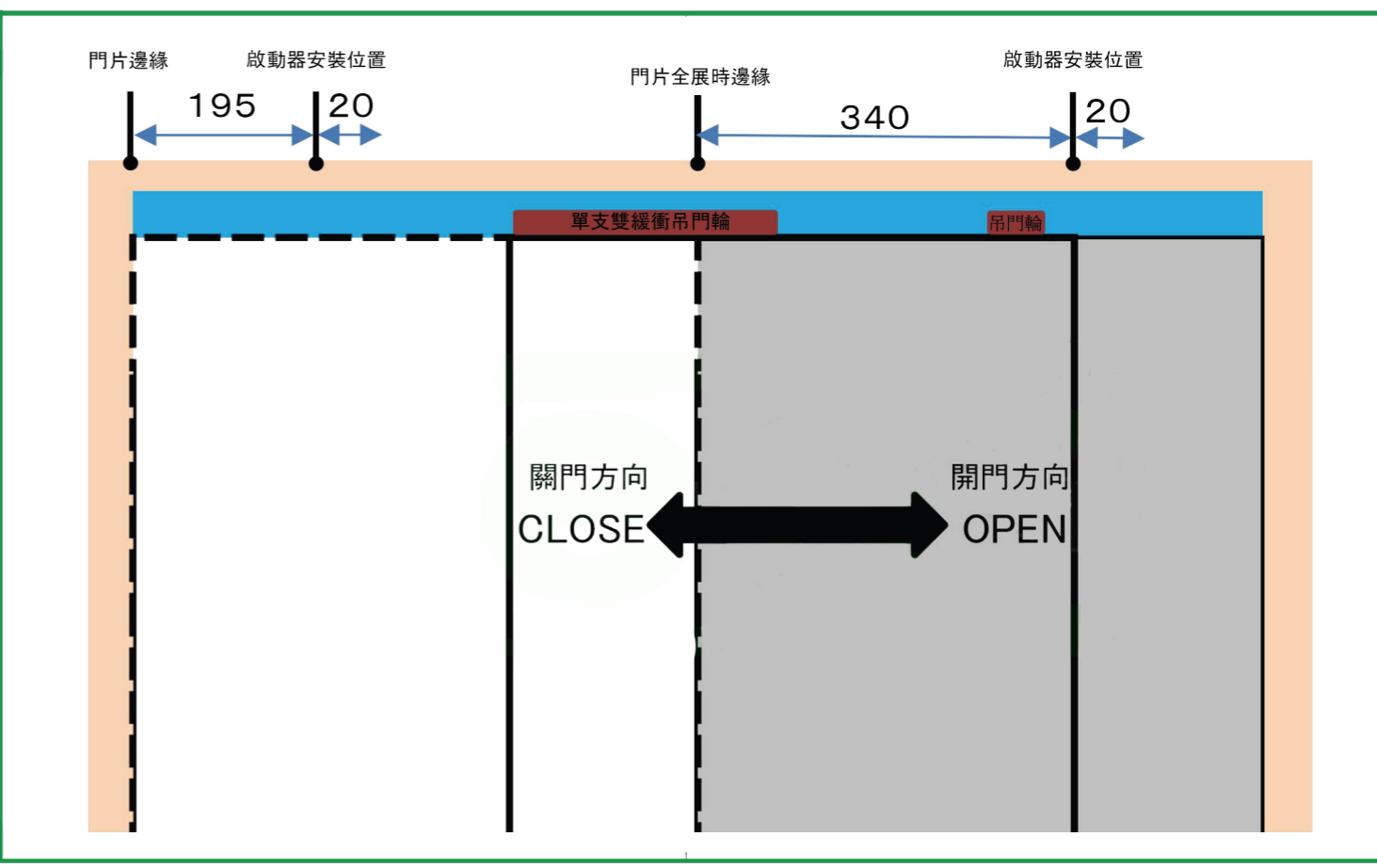
啟動器安裝位置參考示意圖
