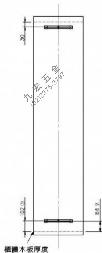
STEP 3: 門板T吧安裝尺寸
