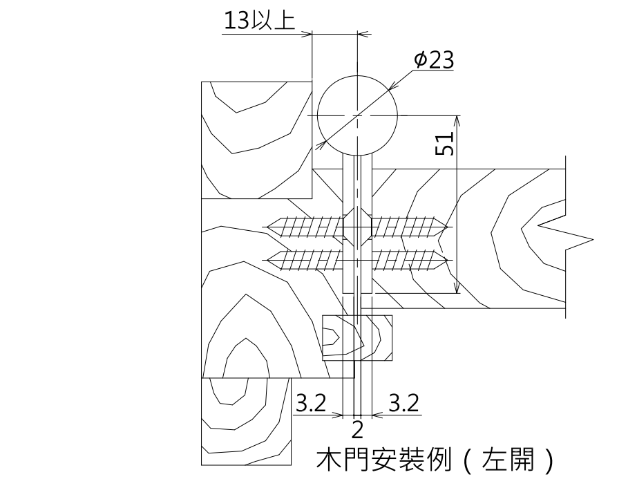
安裝狀態圖
