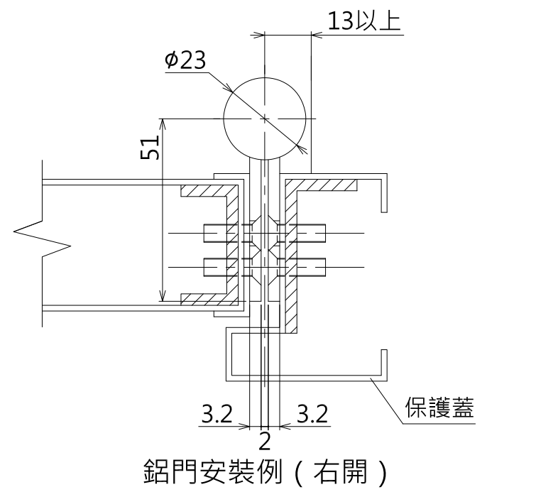
安裝狀態圖
