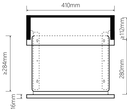
付視圖(打開狀態)
