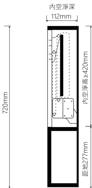
側剖視圖(閉合)
