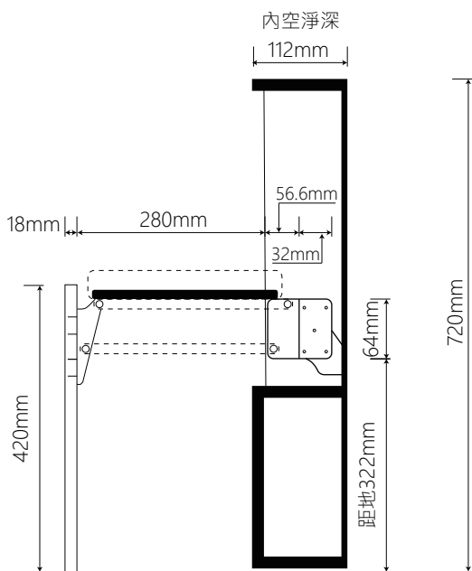
側剖視圖(展開)
