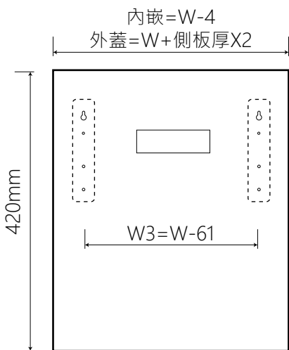
面板孔位圖
